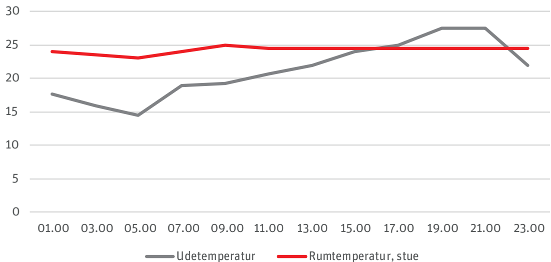
Ude- og indetemperatur med passiv køling
